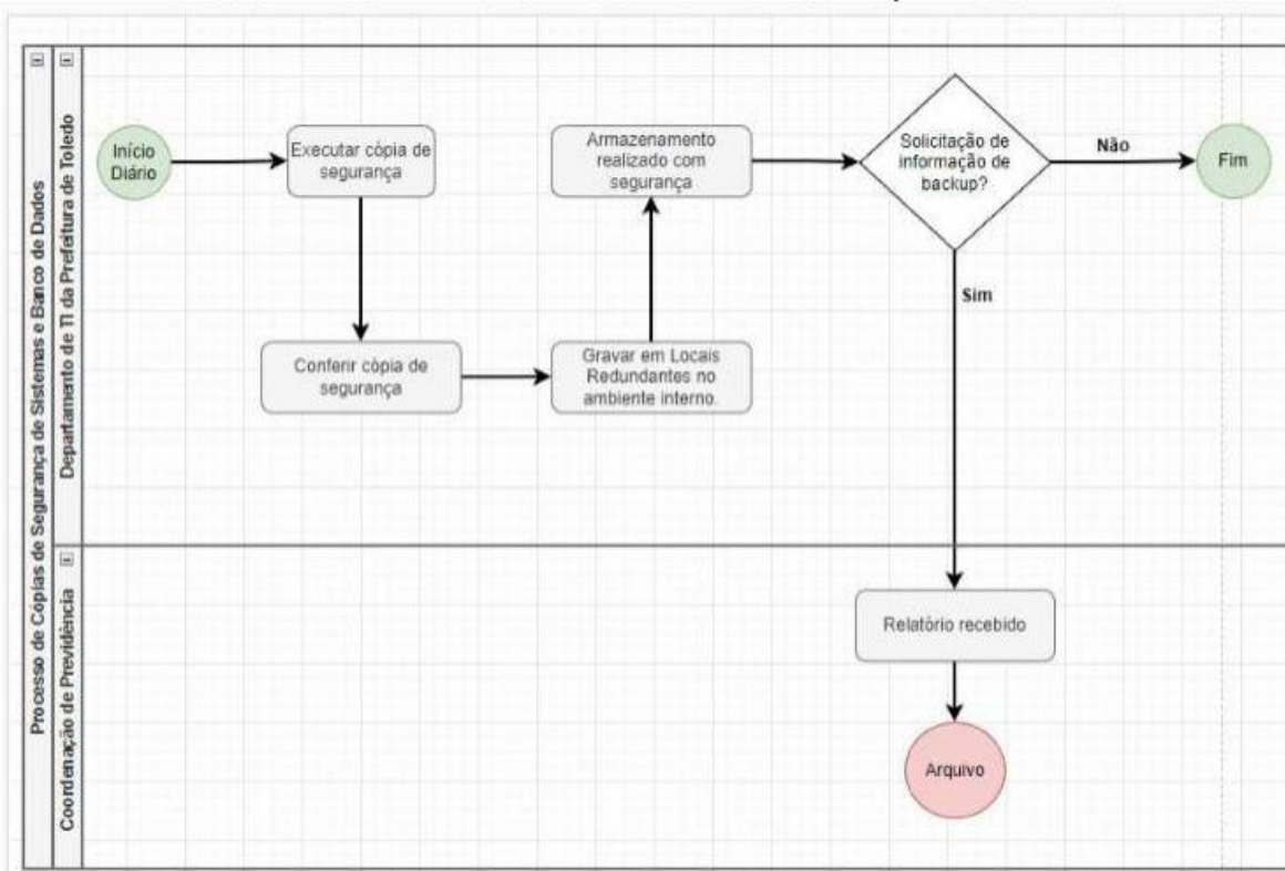
Figura 15 – Procedimentos de Cópias de Segurança de Sistemas e Banco de Dados 22
